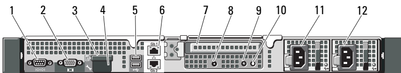
Abbildung 1-4. Anzeigen und Merkmale auf der Rückseite
