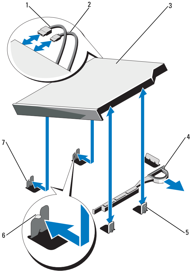
Abbildung 3-17. Optisches Laufwerk ausbauen
