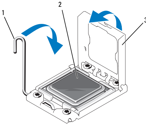
Abbildung 3-24. Installieren eines Prozessors
