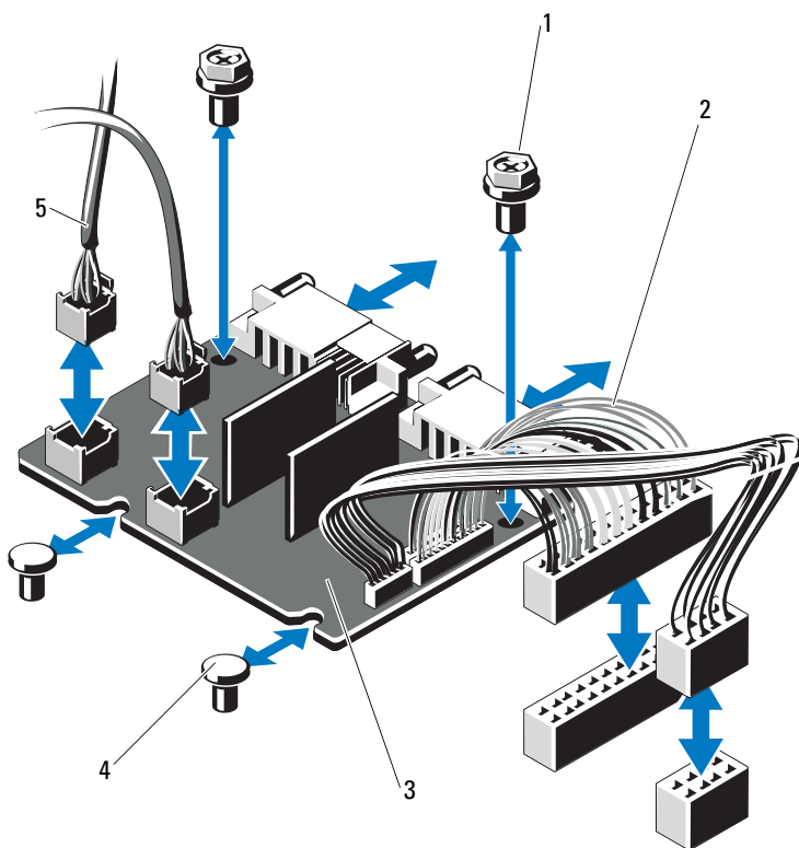
Abbildung 3-29. Stromverteilerplatine
