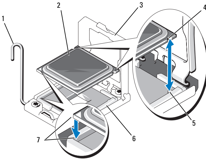
Abbildung 3-23. Ausrichten des Prozessors mit den Sockelpassungen
