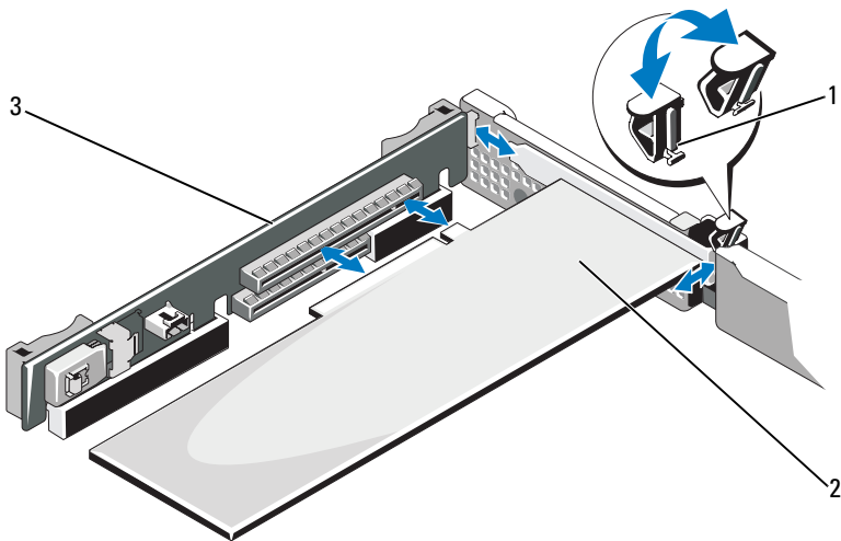
Abbildung 3-9. Erweiterungskarte installieren oder entfernen
