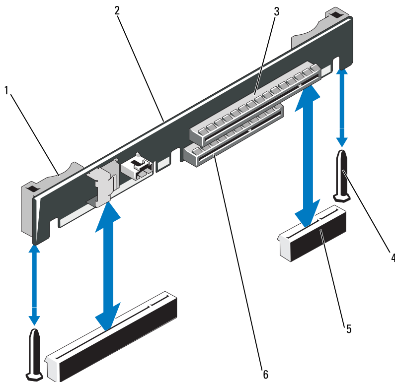
Abbildung 3-11. Erweiterungskarten-Riser installieren oder entfernen
