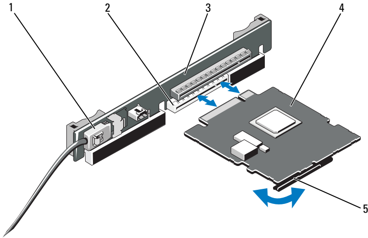
Abbildung 3-10. Integrierte Speichercontrollerkarte installieren
