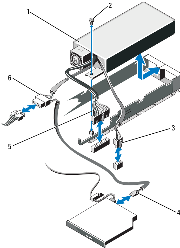
Abbildung 3-8. Nicht-redundantes Netzteil entfernen und installieren
