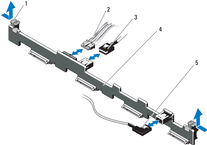
Abbildung 3-28. SAS-Rückwandplatine entfernen und installieren
