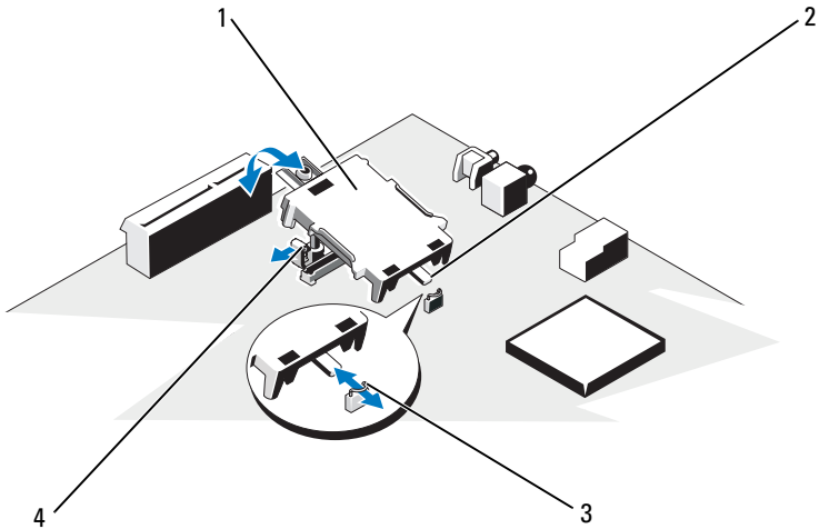
Abbildung 3-14. iDRAC6 Express-Karte (optional) installieren oder entfernen
