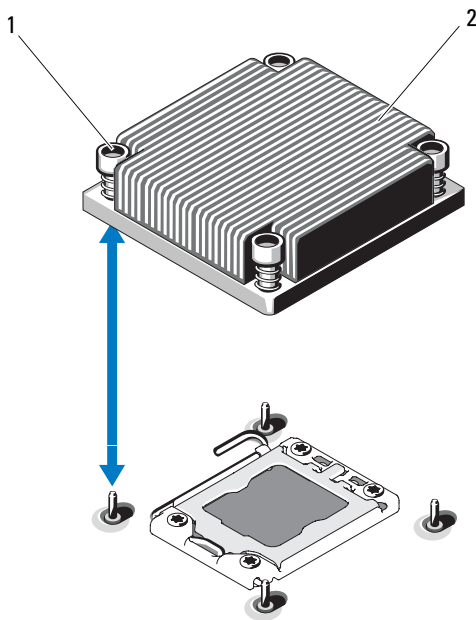
Abbildung 3-20. Kühlkörper installieren und entfernen
