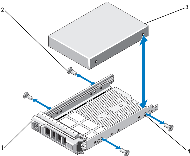
Abbildung 3-6. Festplatte im Laufwerkträger installieren
