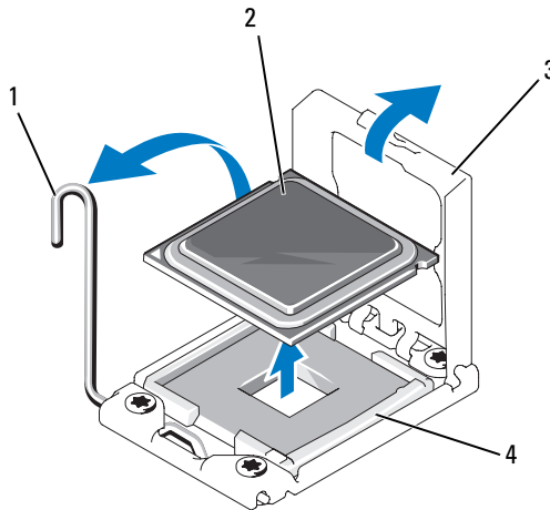
Abbildung 3-21. Entfernen eines Prozessors
