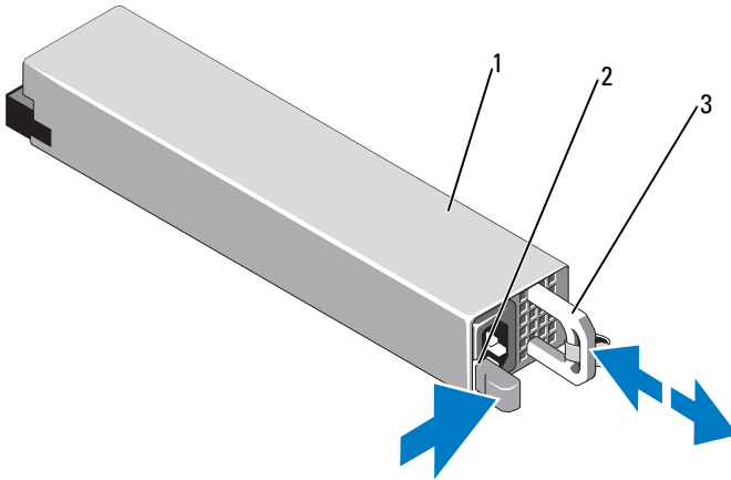
Abbildung 3-7. Redundantes Netzteil entfernen und einsetzen
