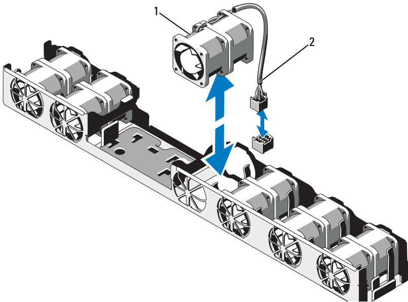
1 Lüfter 2 Stromversorgungskabel
