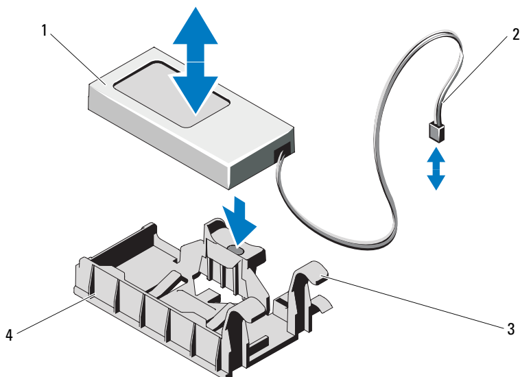
Abbildung 3-18. RAID-Akku entfernen und installieren
