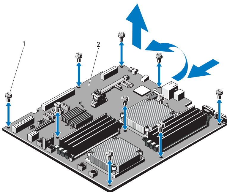
Abbildung 3-30. Systemplatine entfernen und installieren
