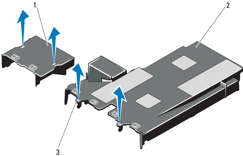
Abbildung 3-13. Kühlgehäuse der Systemplatine installieren und entfernen
