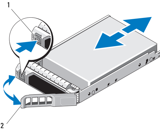
1 Entriegelungstaste 2 Griff des Festplattenträgers
