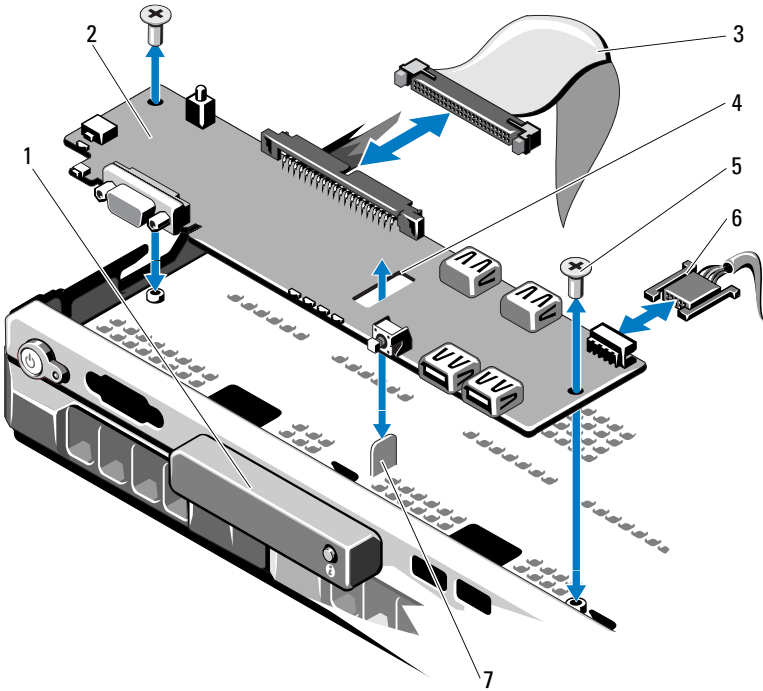
Abbildung 3-26. Bedienfeldplatine entfernen – LED (optional)
