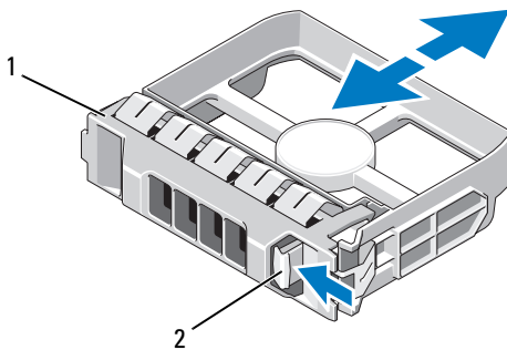
1 Laufwerkplatzhalter 2 Entriegelungshebel
