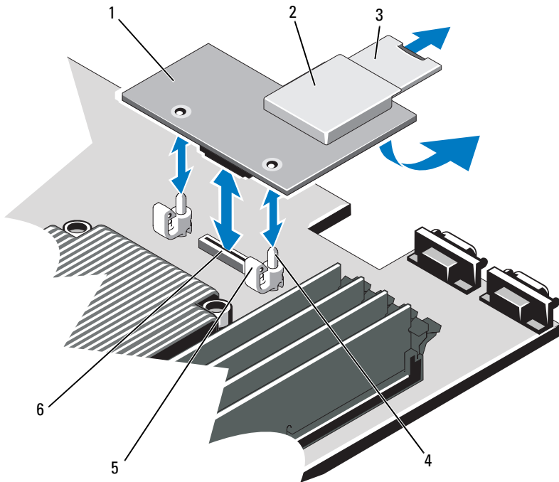
Abbildung 3-15. iDRAC6 Enterprise-Karte (optional) installieren oder entfernen
