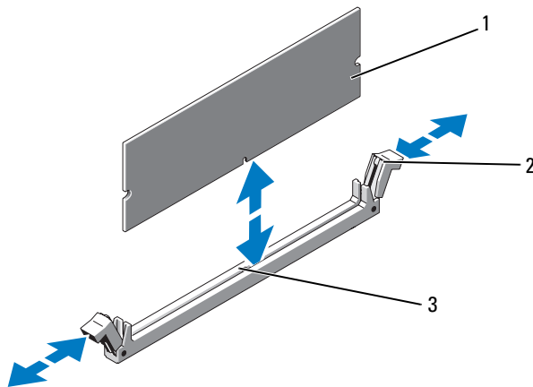
Abbildung 3-19. Speichermodul installieren und entfernen
